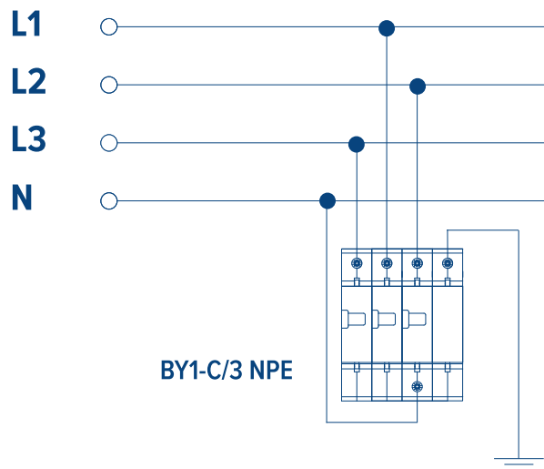
Sieć typu TT
