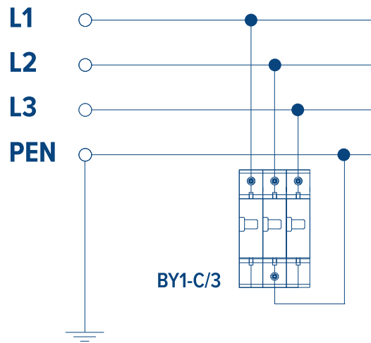
Sieć typu TN-C
