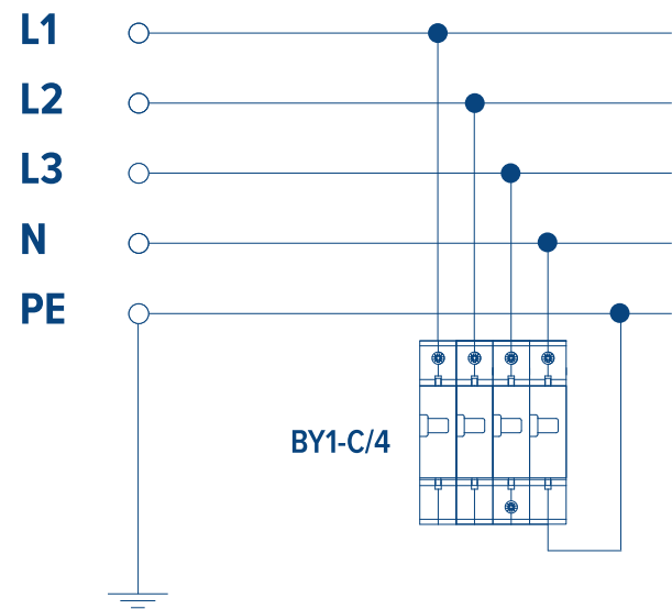
Sieć typu TN-S
