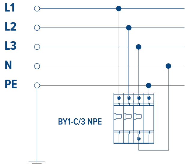
Sieć typu TN-S
