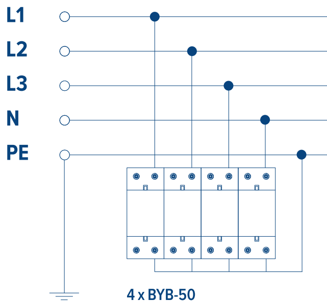
Sieć typu TN-S
