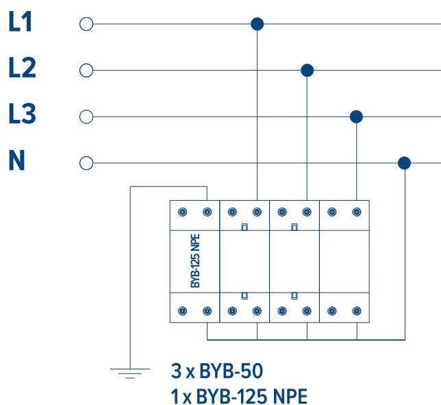
Sieć typu TT
