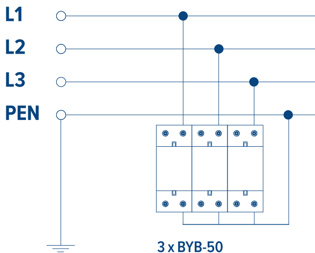
Sieć typu TN-C
