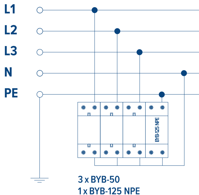
Sieć typu TN-S
