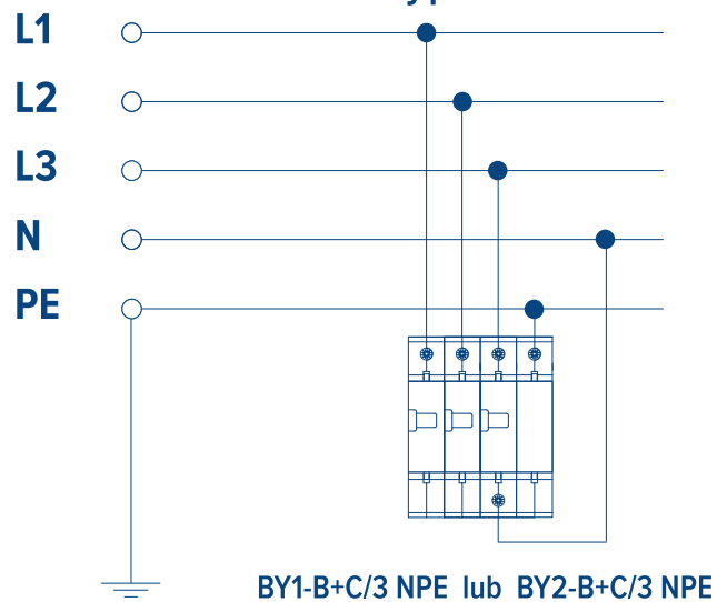
Sieć typu TN-S
